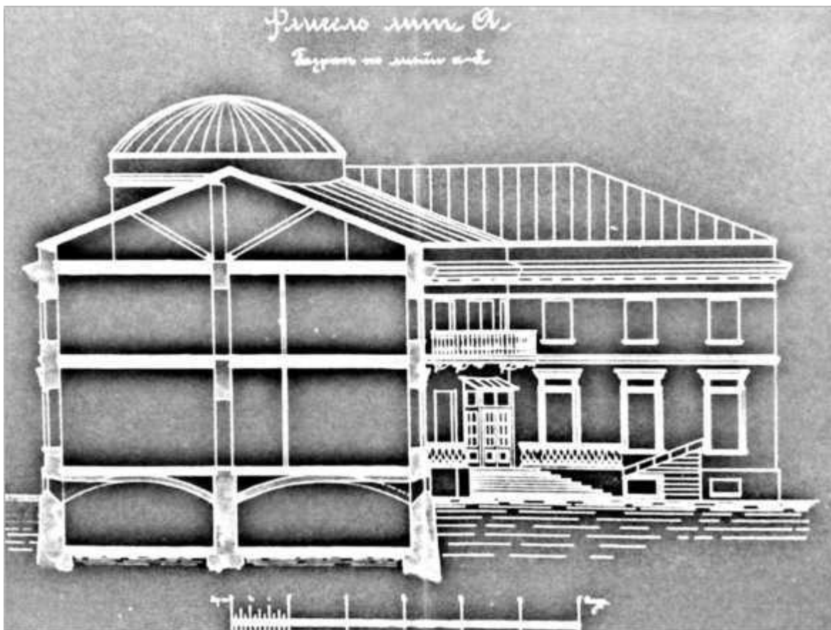
Чертежи Малоохтинской больницы в Петербурге. Поперечный разрез корпуса, расположенного вдоль Охты. Синька. Цит.: РГИА Ф. 768. Оп. 2. Д. 1231*. 1880-е гг.
