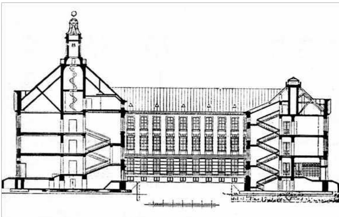
Здание Главного Гидрографического управления. Разрез. Цит.: Малеин Н.И. Здание Главного Гидрографического управления (пояснительная записка и чертежи). Пг., 1916 г.
