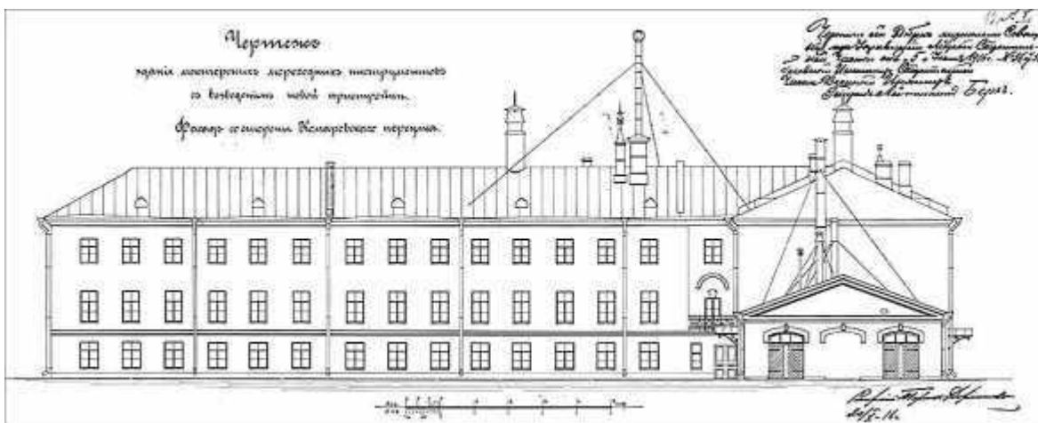
Чертеж здания мастерской мореходных инструментов с возведением новой пристройки. Цит.: РГА ВМФ. Ф. 404. Оп. 1. Д. 787. Л. 12
