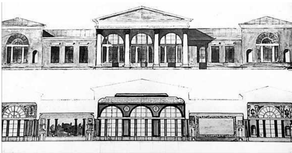
Дача Безобразова в имени «Екатериновка», станция «Жерновка». Обмерный чертеж. Арх. А. Соколов. 1924 г. Цит.: Отдел хранения изобразительных памятников. ГМИ Санкт-Петербурга
