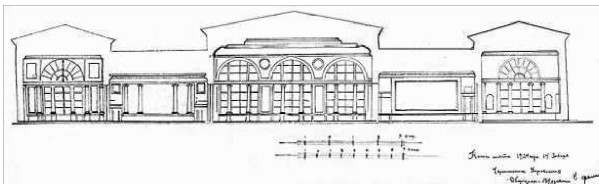
Дача Безобразовых. Продольный разрез. Н. Фомин. 1923–1925 гг. Цит.: ЦГА. Ф. 2555. Оп. 1. Д. 1181
