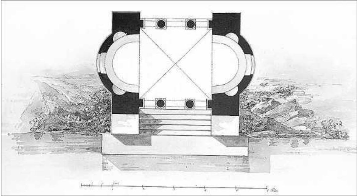
Усадьба М.И. Донаурова. Павильон-пристань. План. Дж. Кваренги. Сер. 1790-х гг. © ГЭ. Сектор рисунков отдела западноевропейского изобразительного искусства. Фото С.В. Суетовой, К.В. Сияевского. 2016 г.
