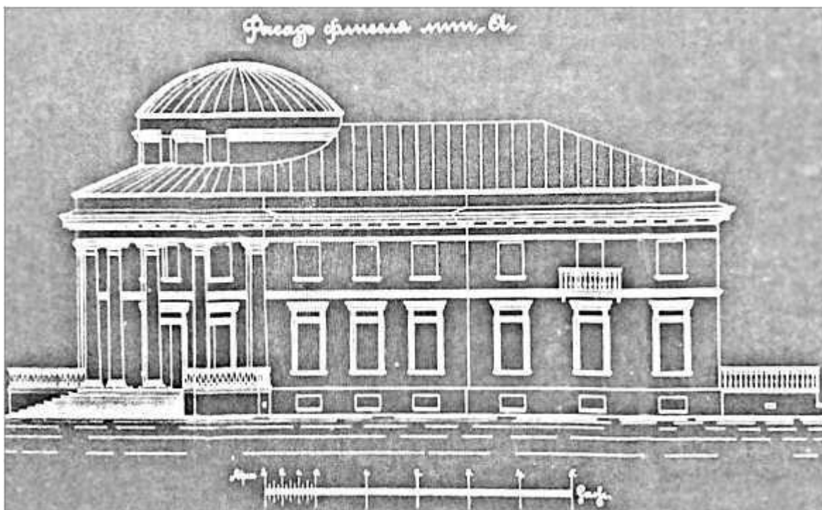
Чертежи Малоохтинской больницы в Петербурге. Фасад со стороны Охты. Синька. Цит.: РГИА Ф. 768. Оп. 2. Д. 1231*. 1880-е гг.
